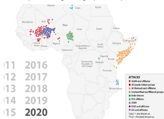
شکل (۱): نقشه حملات گروه‌های افراطی اسلامی در قاره آفریقا (۲۰۱۶-۲۰۲۰)
